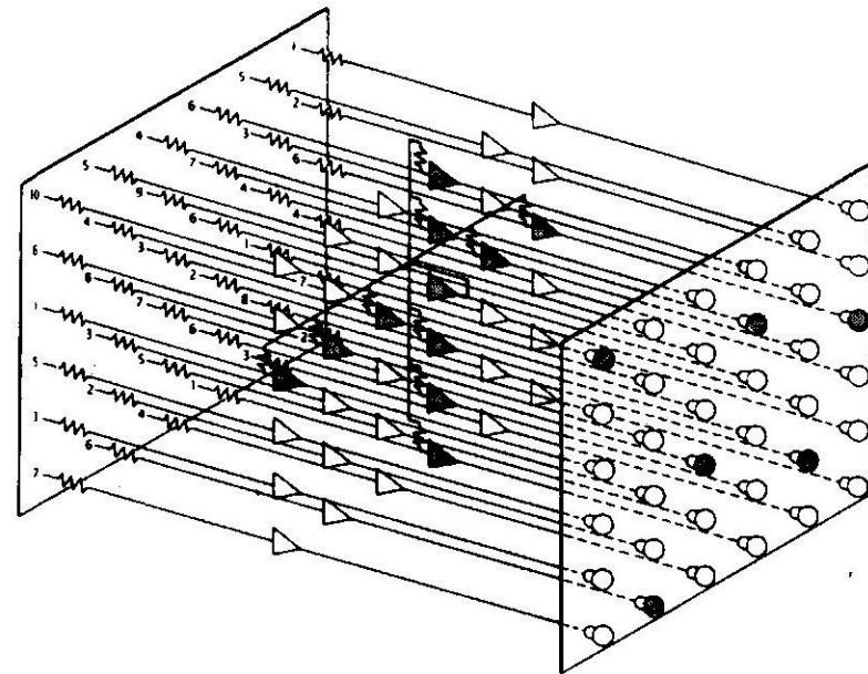
Figura 5. Red de Hopfield. Un circuito de optimización para resolver el problema de asignación de tareas. Consiste en una red de n -flops interconectados. Los amplificadores de cada hilera y columna están enlazados por conexiones inhibitorias que imponen la restricción de que sólo un amplificador por hilera o columna pueda hallarse en estado +1. Como cada uno de los 36 amplificadores de esta red inhibe a otros 10 amplificadores, hay 360 conexiones en total. El diagrama presenta las conexiones de uno de los amplificadores. Los amplificadores reciben entradas de corriente proporcionales a las tasas de reducción. Los amplificadores que corresponden a la mejor solución – la combinación de entradas [inputs] que suman el total mayor – emiten un +1 y el resto emite un 0. Las emisiones [outputs] pueden controlar un panel, en este caso un conjunto de bombillas eléctricas. (Fuente: Hopfield y Tank, "Collective Computation in Neuronlike Circuits", Scientific American , diciembre 1987)
